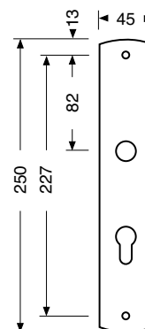
KZS für Zylinder- überstände 9 – 11 mm.
