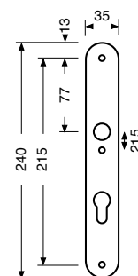
KZS für Zylinder- überstände 8 – 13 mm.
